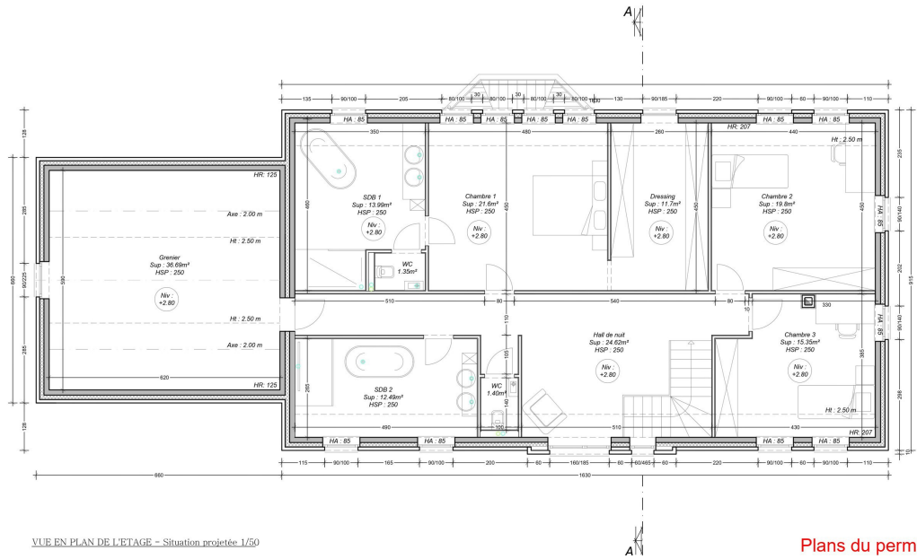
VUE EN PLAN DE L'ETAGE – Situation projetée 1/50
