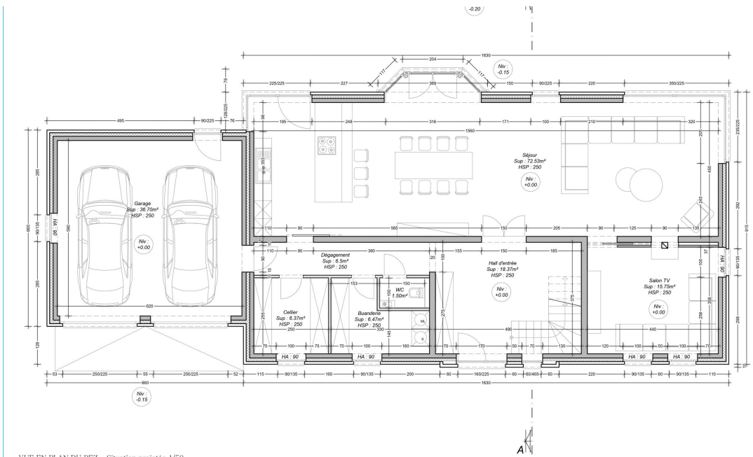
VUE EN PLAN DU REZ – Situation projetée 1/50
